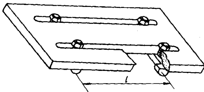
图 8 调整中心距
