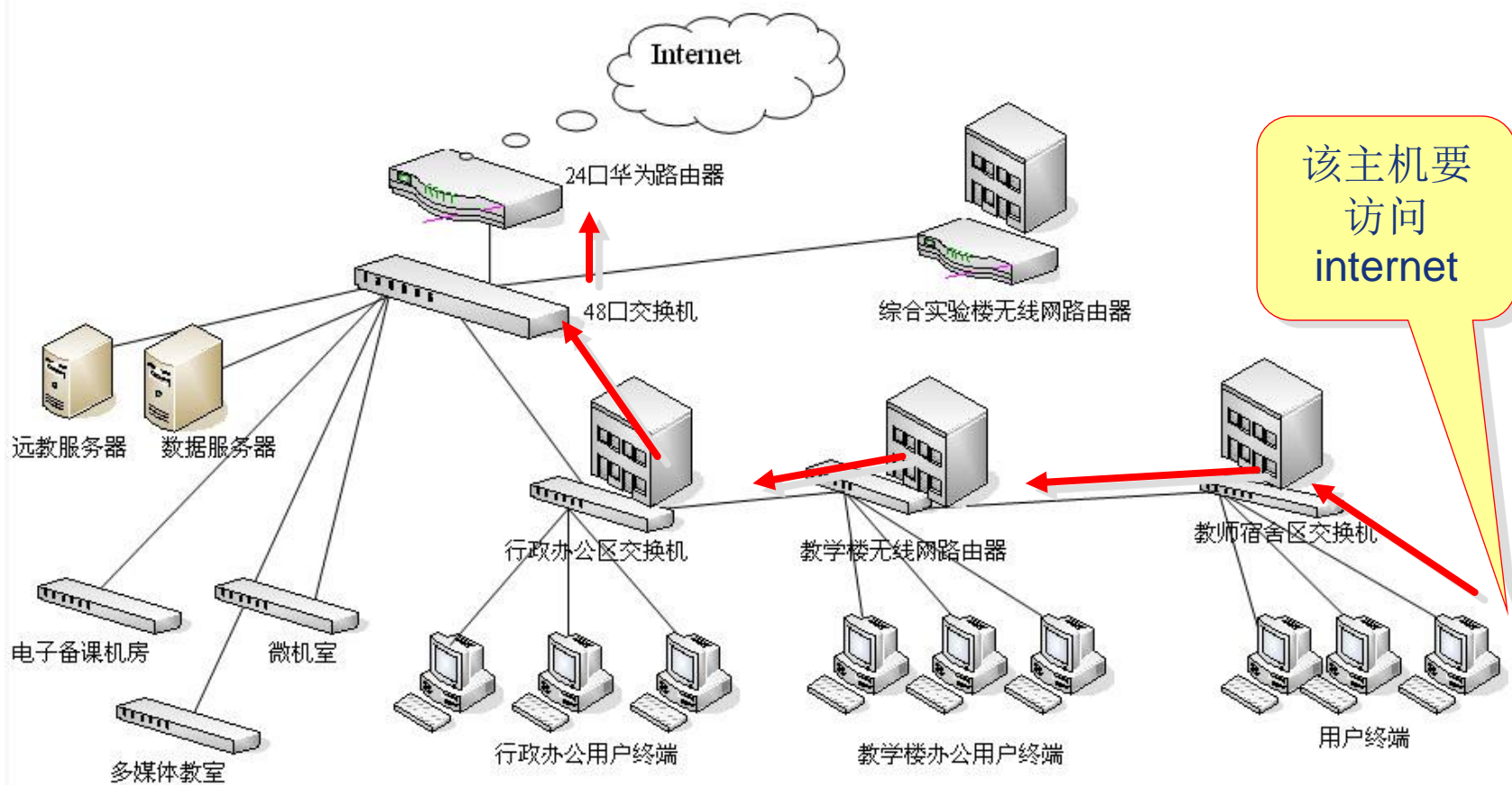
杨井中学局域网网络拓扑结构图
