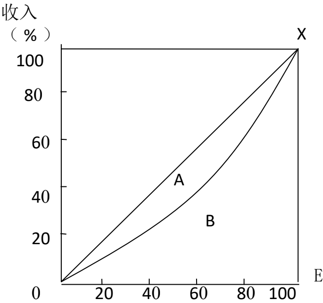
图 7-17 洛伦茨曲线
